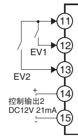
事件输入/控制输出2规格
