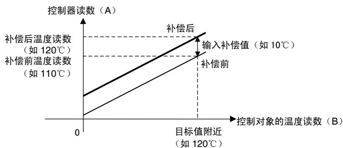
图 2 1 点温度输入补偿
