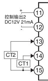
控制输出/CT2规格
