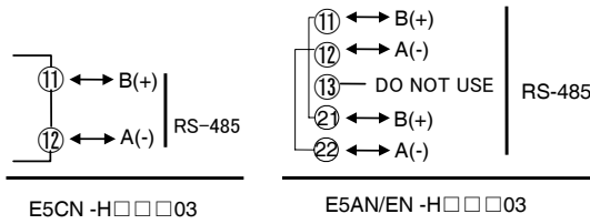
通信单元接线图
