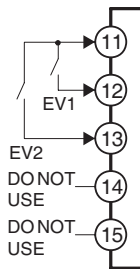
事件输入规格
