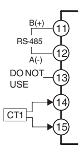
通信 (RS-485) / CT规格
