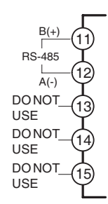
通信 (RS-485) 规格
