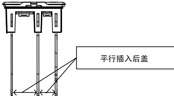
E5CN-H 的下侧图
